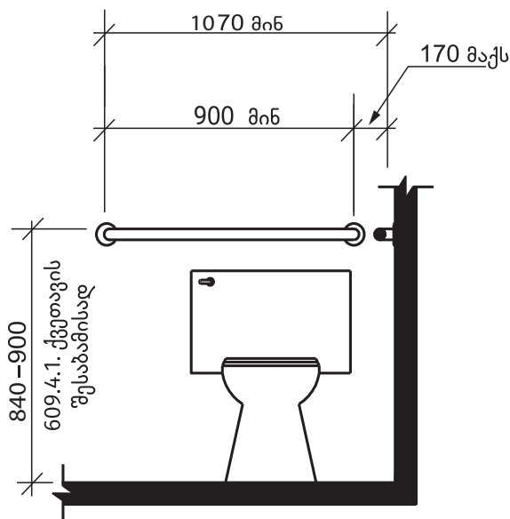
სურათი 604.5.2 ხელმოსაჭიდი ძელი უნიტაზის უკან მდებარე კედელზე
