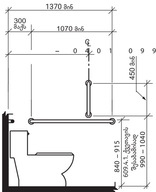
სურათი 604.5.1 უნიტაზთან დამონტაჟებული ხელმოსაჭიდი ძელი გვერდითა კედელზე
